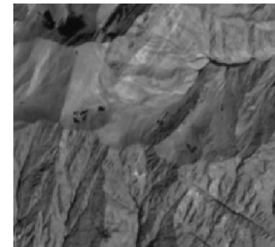
SWIR
