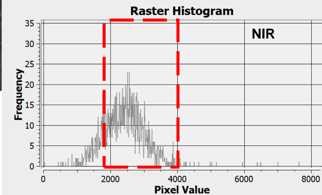
B8 (NIR)
