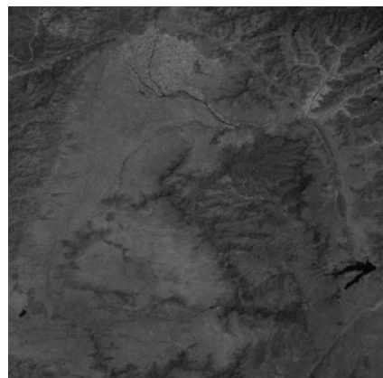
B8 (NIR)
